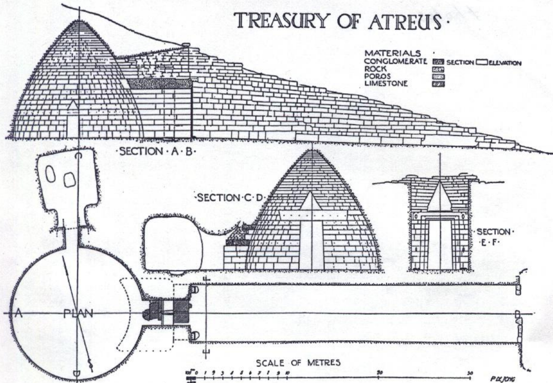
Fig. 15. 'Treasury of Atreus', Mycenae
