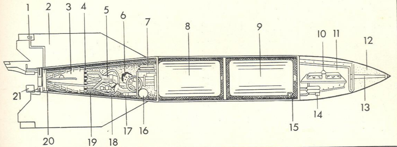
Esquema de la bomba V-2: 1) aletas exteriores de control; 2) aletas estabilizadoras; 3) cámara de combustión; 4) ignitores; 5) sistema de circulación de alcohol; 6) mecanismos de turbinas y bombas; 7) recipientes de aire; 8) tanque de oxígeno líquido; 9) tanque de alcohol; 10) equipo radio director; 11) compartimiento de control; 12) carga explosiva; 13) mecanismo detonador; 14) recipiente de nitrógeno; 15) giróscopo; 16) tanque de peróxido de hidrógeno; 17) tanque de permanganato; 18) bomba para la distribución de oxígeno; 19) tuberías de enfriamiento por alcohol; 20) servomotores hidráulicos; 21) aletas interiores de control.
